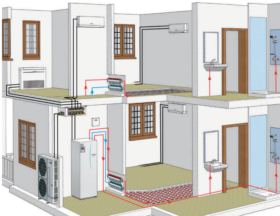
SCHEMA SMALL Y CON ECODAN
